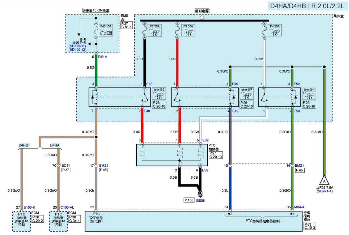
空调控制系统(自动)(6)
